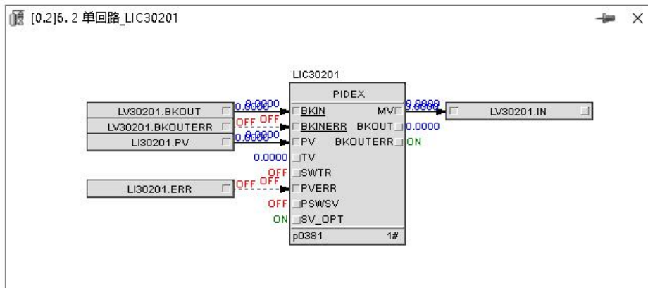
图 1- 9 逻辑图
